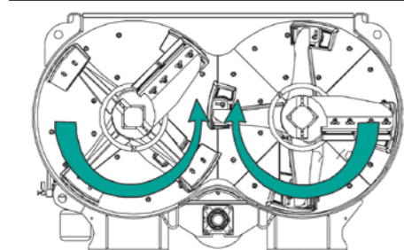
Rotazione degli assi di mescolazione sincronizzata e contrapposta
